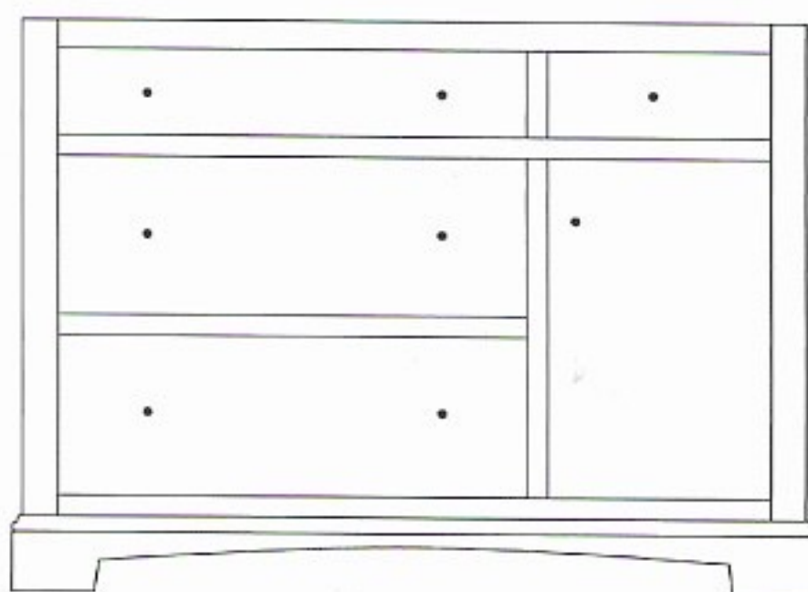
DSB-247 47¼"w 34½"h 24½"d w/4 drawers, 1 door
